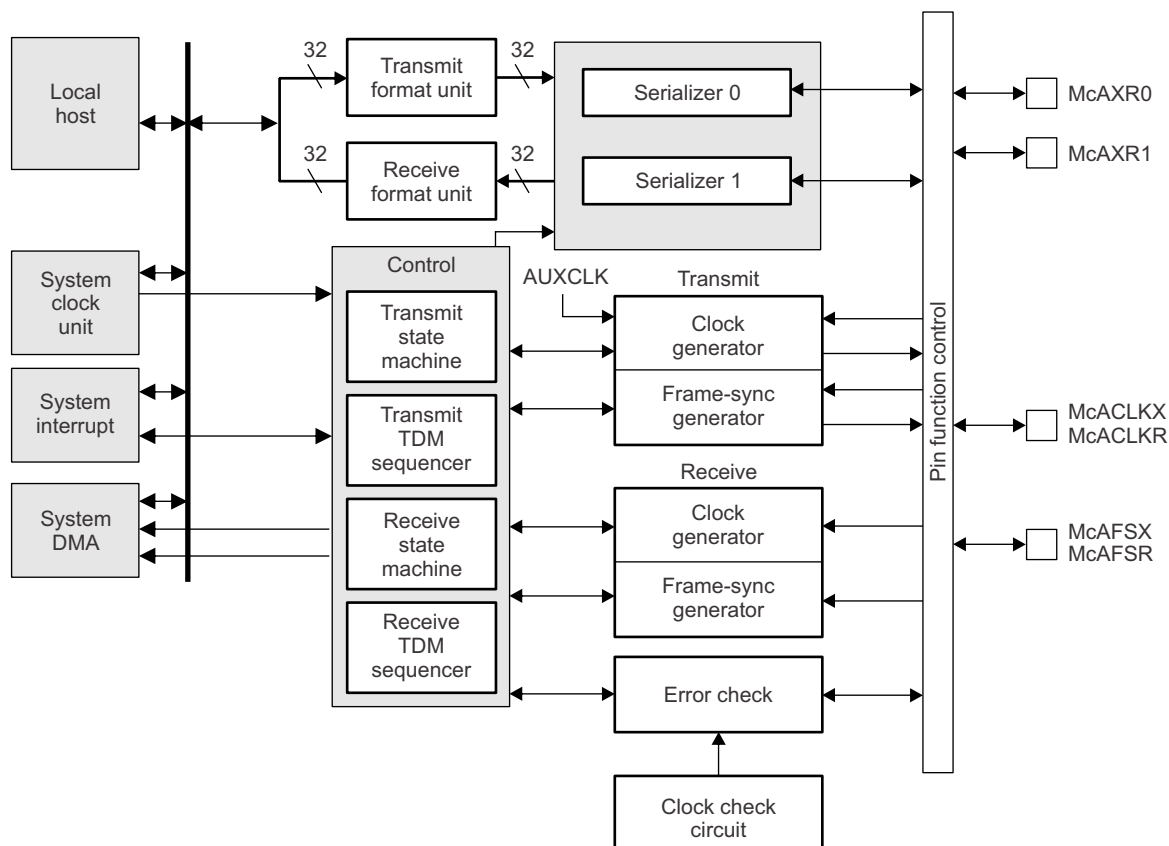
Figure 12-2. MCASP Module
